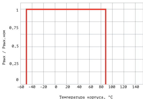
График зависимости выходной мощности от температуры корпуса при использовании радиатора.
